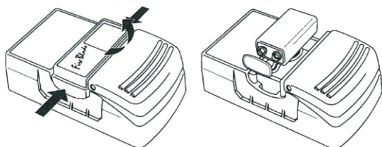
1 / ボディ上面の電池カバーを両サイドから押しつつフットペダル側の方から引き上げるように外します 2 / 新しい電池に交換します。
