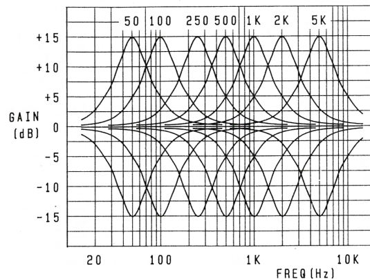
ベースEQの周波数特性
